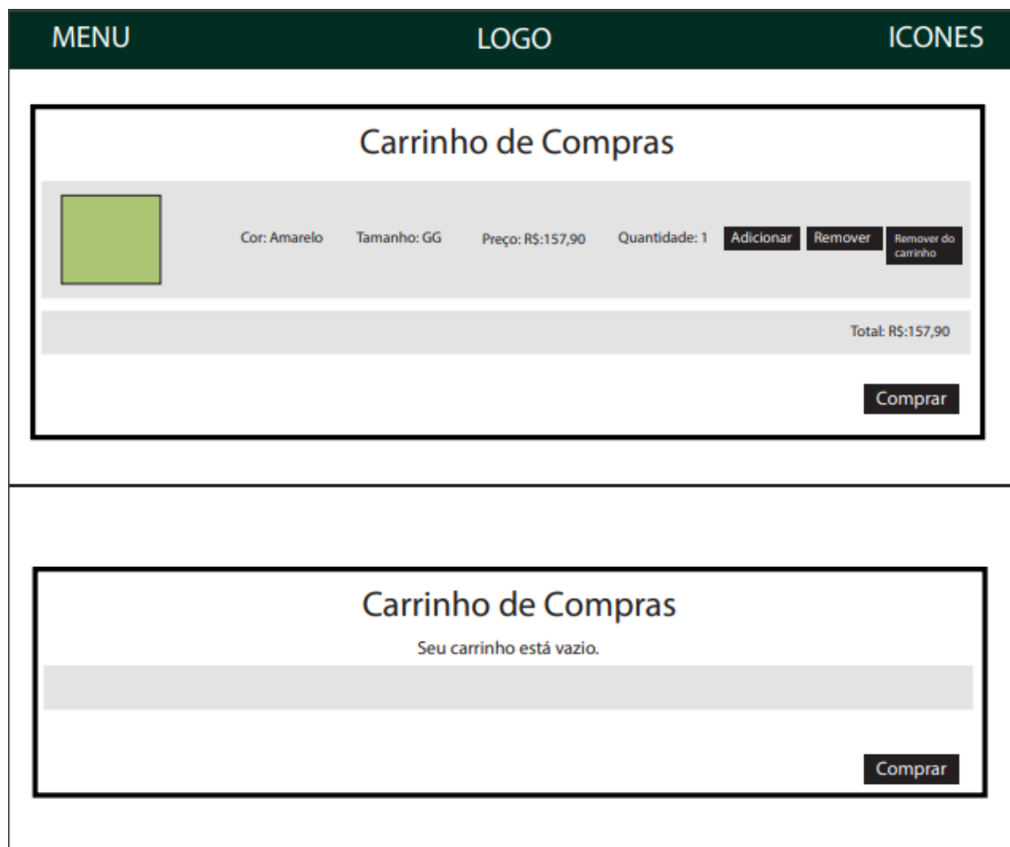
Figura 12 – Boneco Página Carrinho de compras
