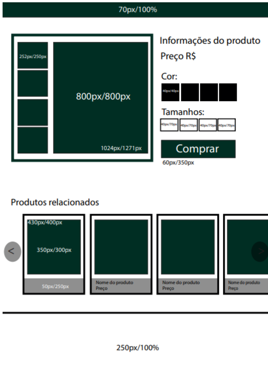
Figura 15 - Layout das Páginas Individuais
