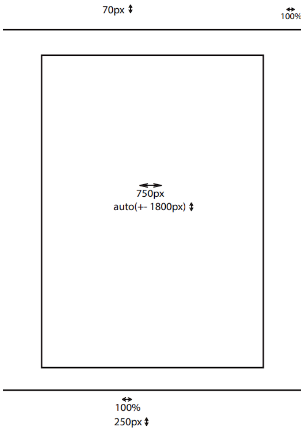
Figura 19 - Layout da Página Termos de Uso
