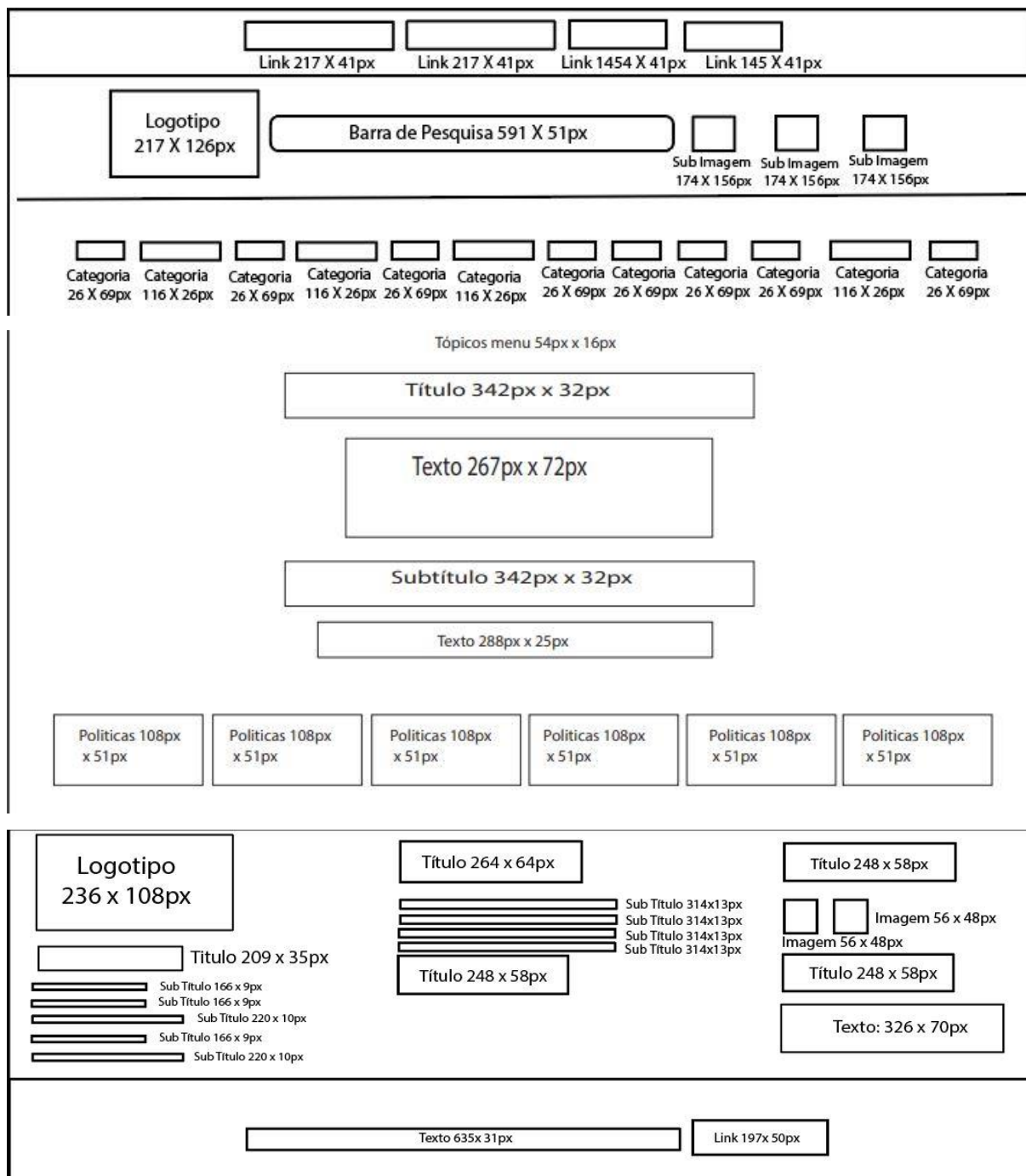
Figura 43 - Layout da Página Sobre (Peach)
