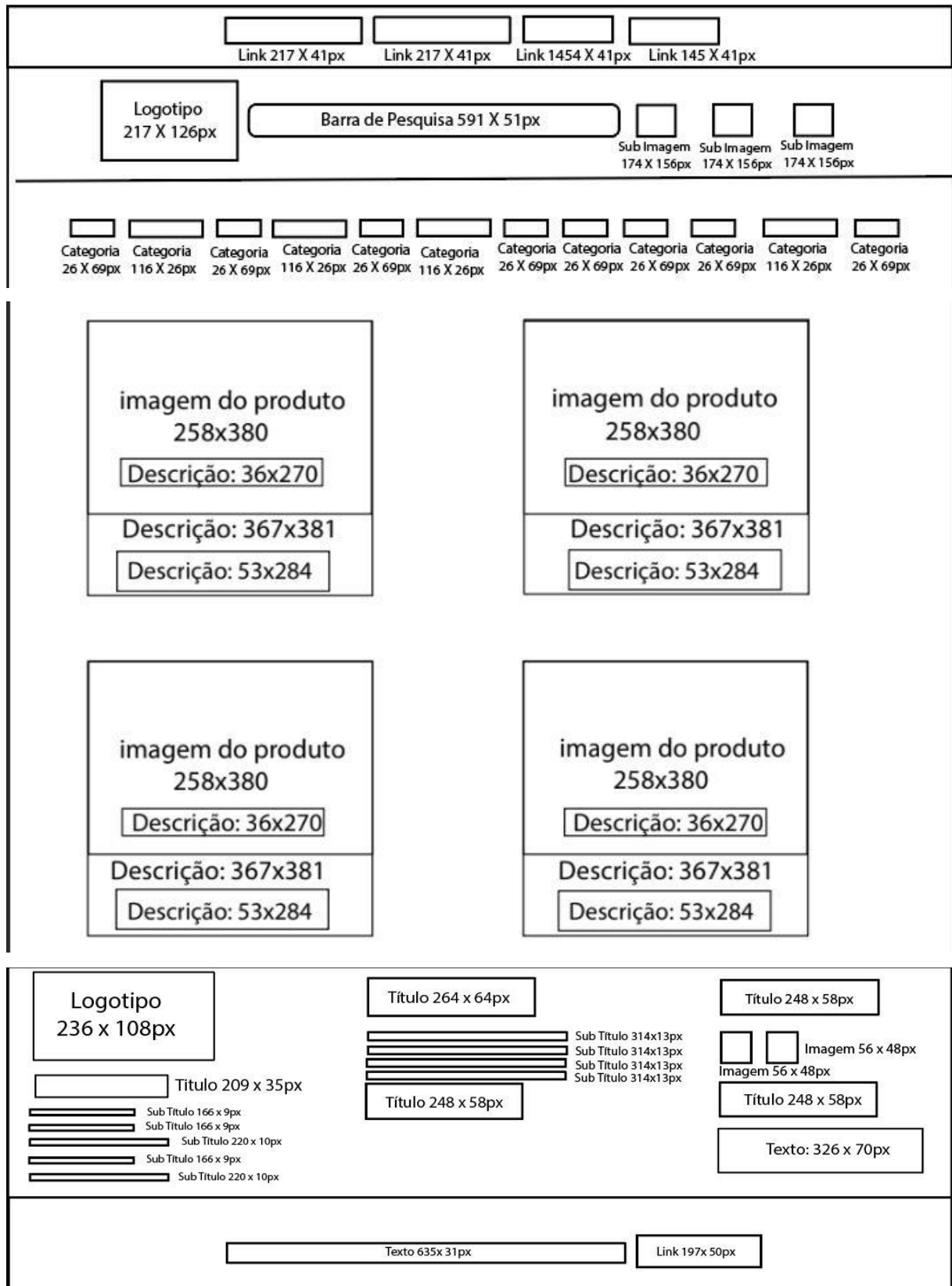
Figura 36 - Layout da Página de Favoritos
