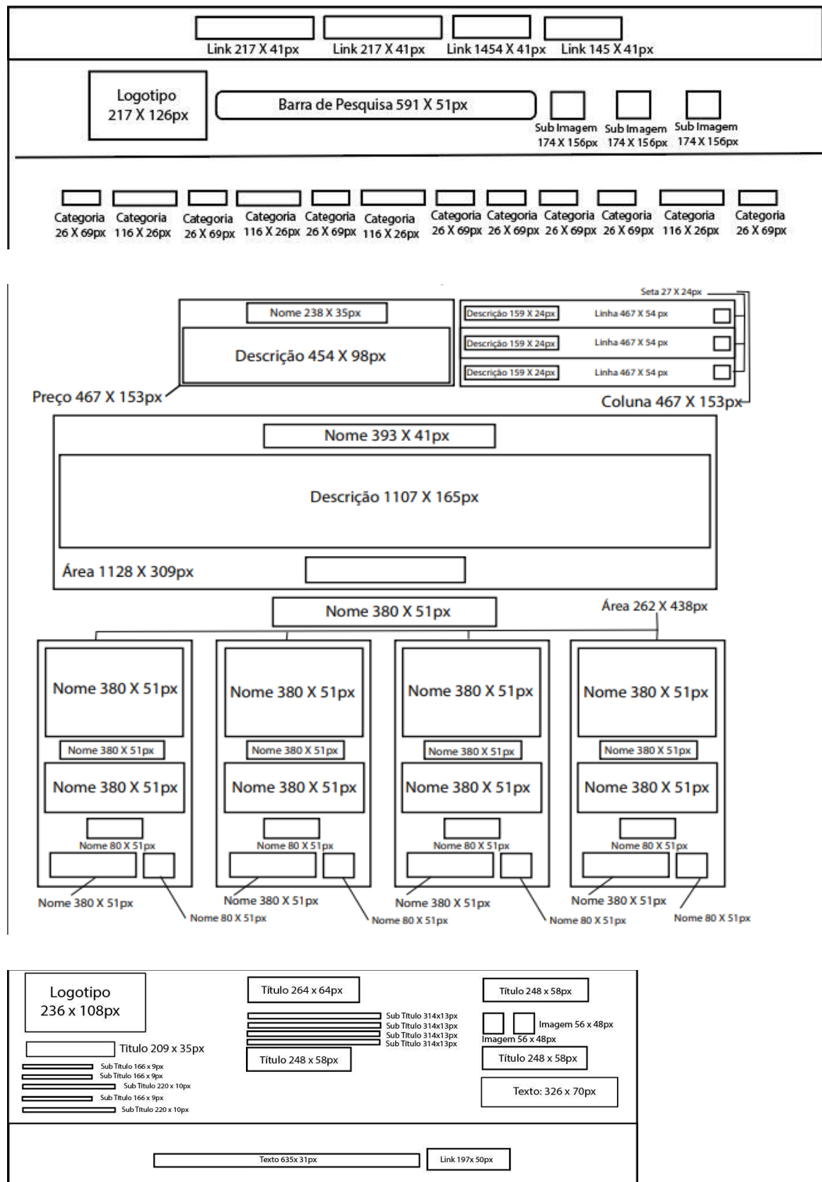
Figura 29 - Layout da Página Individual
