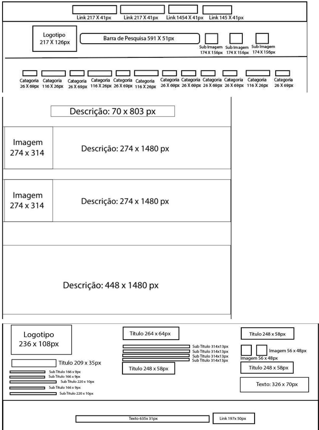
Figura 38 - Layout da Página de Carrinho
