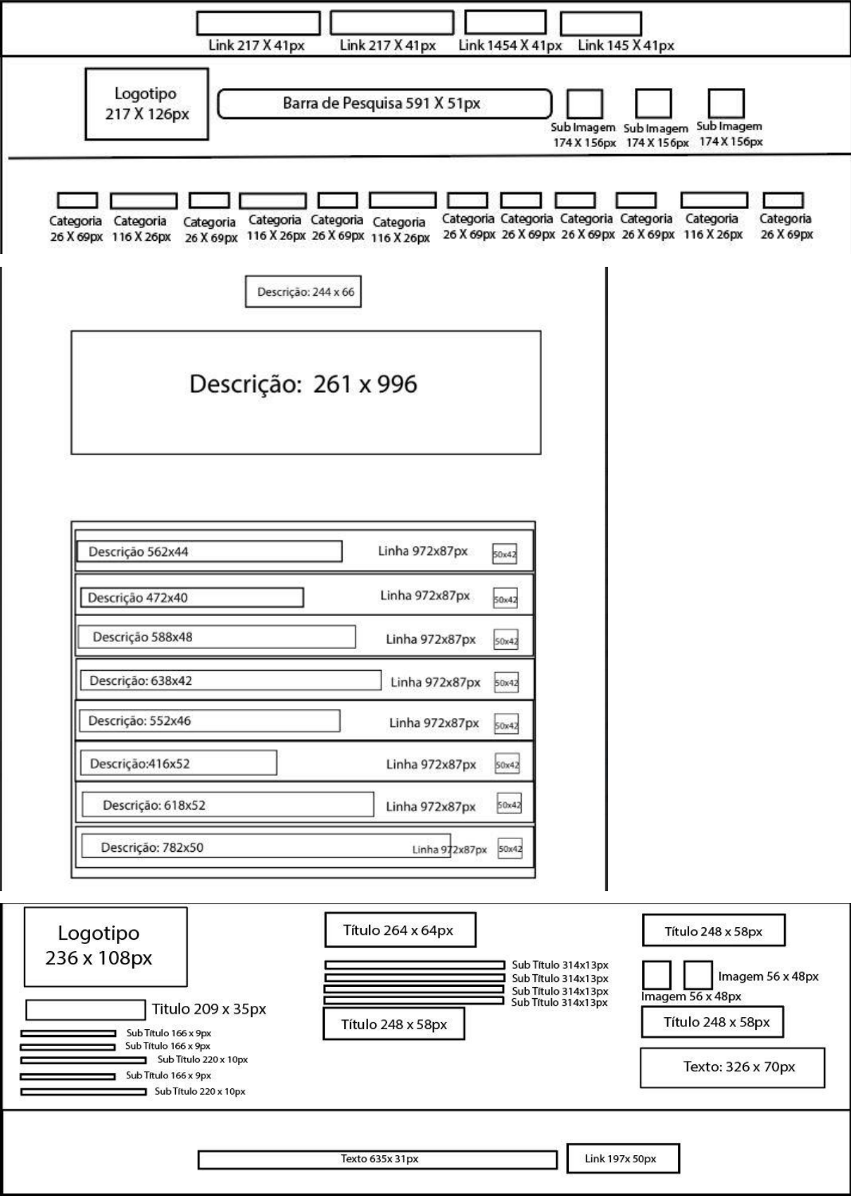
Figura 33 - Layout da Página de Ajuda
