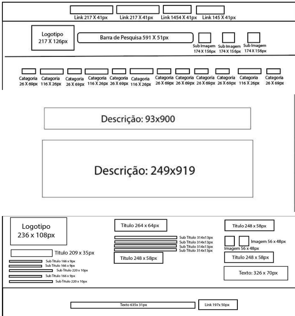
Figura 32 - Layout da Página de Pagamento
